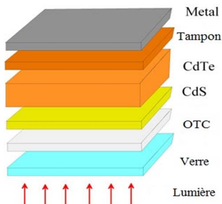
Coupe de cellule photovoltaïque CdTe (adapté d'après SSE 1 )
