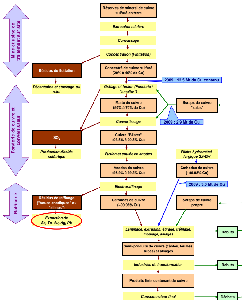
Position de la production des boues anodiques à tellure et autres éléments dans le processus de production de cuivre par pyrométallurgie
